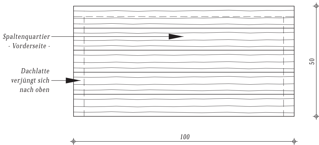
- Vorderansicht - 1 : 10
