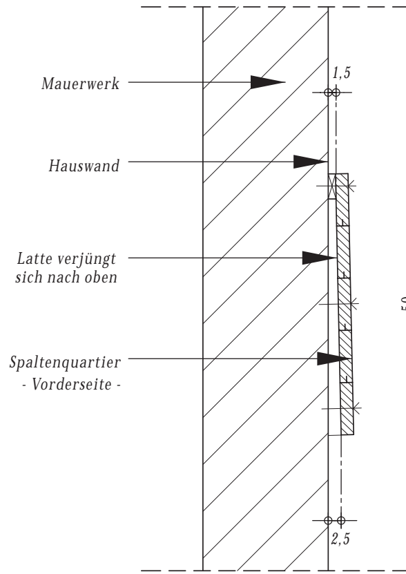
- Querschnitt - 1 : 10
