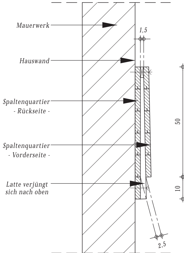
- Querschnitt - 1 : 10
